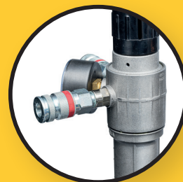
2 Qualitätskupplungen ARO 210
